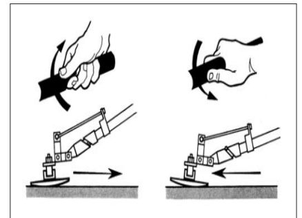
Verstellbarer Anstellwinkel
