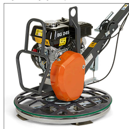
Poignée de réglage des pâles
