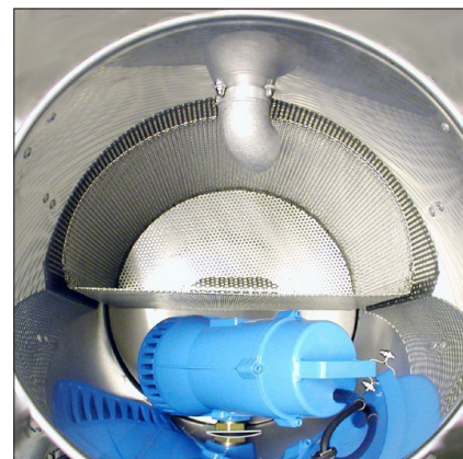
Integrierte Pumpe und Grobsieb
