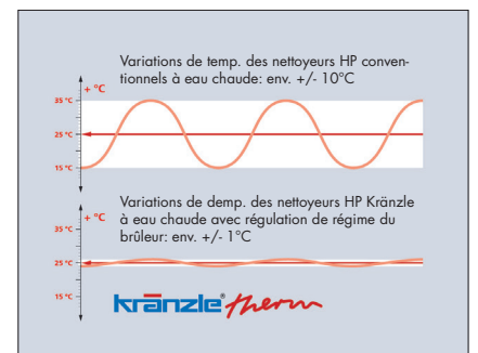
Régulation thermostatique
