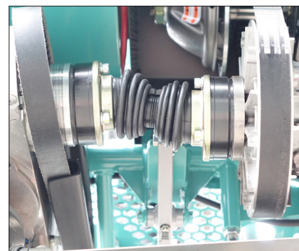
Variomatik-Kupplung
