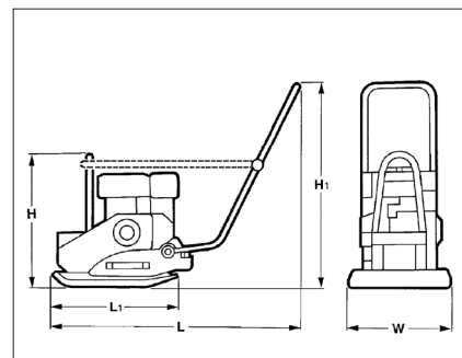
Mit Transportgriffe und Transporträder (Standard)
